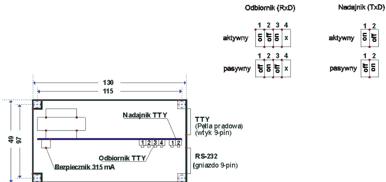
Rys 2 Wybór zasilania
